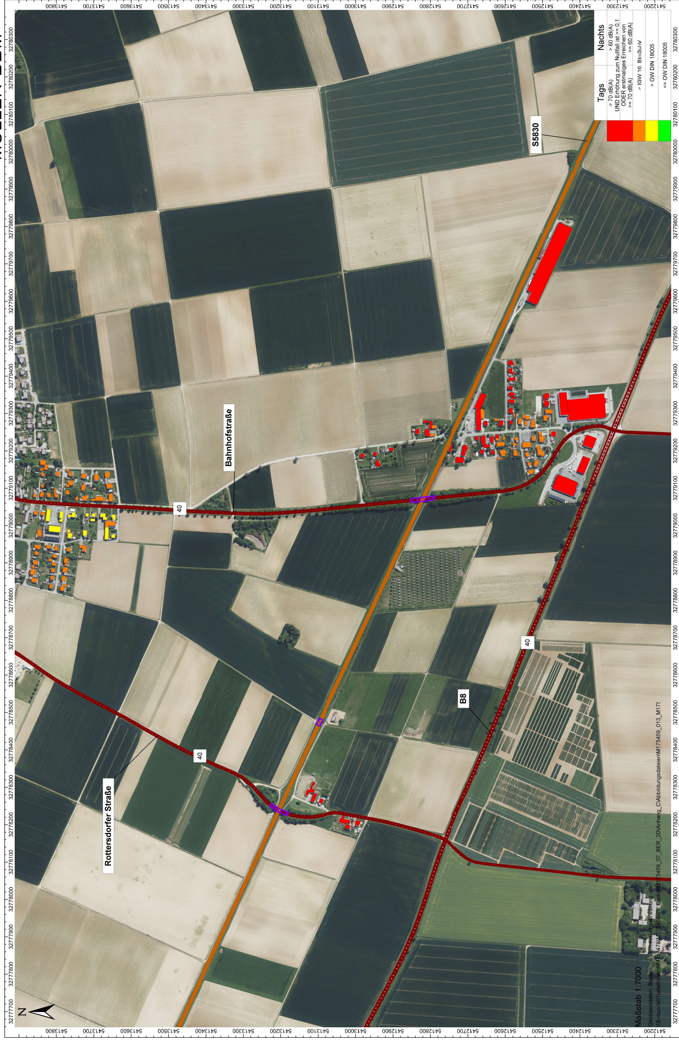
Abbildung C7: Untersuchungsbereich Stephansposching - Kennzeichnung nach Orientierungswerten (OW), Immissionsgrenzwerten (IGW) sowie Zumutbarkeitsschwellen
